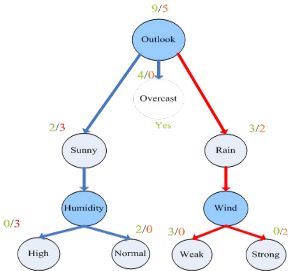
图 1: 决策树算法模型
