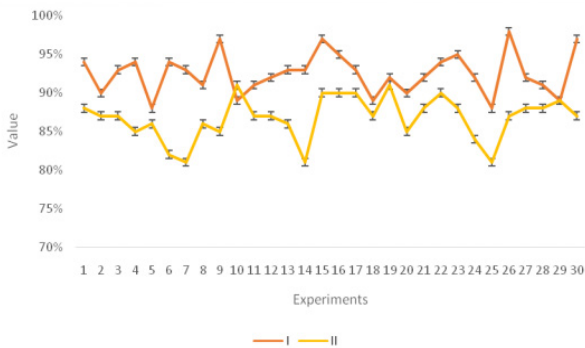
图2：准确率对比
