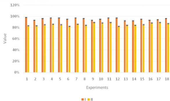
图3：稳定性对比
